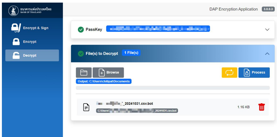
รูป หน้าจอสำหรับ Decrypt ไฟล์
